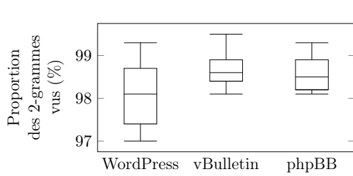
FIGURE 5 – Boîte à moustaches des bigrammes vus pour les trois CMS considérés. Nous montrons dans chaque cas les valeurs minimum et maximum (moustaches), le premier et troisième quartiles (boîte) et la médiane (ligne horizontale).
