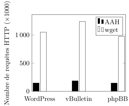
FIGURE 4 – Nombre total de requêtes HTTP utilisées pour crawler le jeu de données
